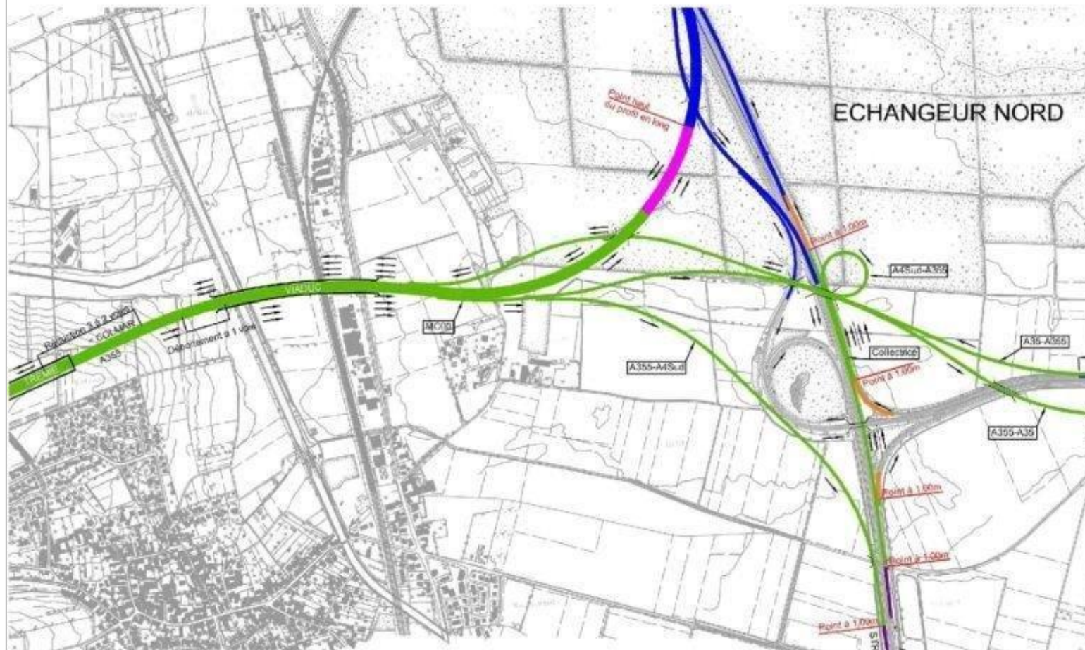
Figure 4 : Noeud autoroutier « Nord » : A355/A35/A4 à Vendenheim / Eckwersheim / Brumath / Geudertheim
